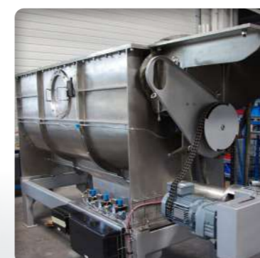
► Entraînement par chaîne du mobile d'agitation
