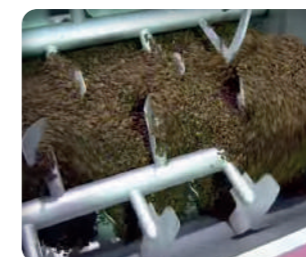
2 Mélangeur à double arbre à pales
