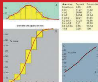
Curva granulométrica
